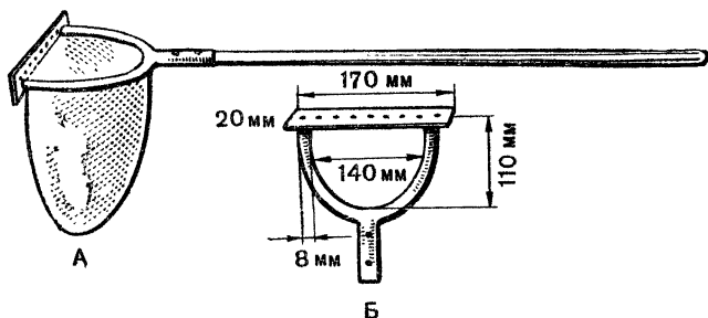
Рис. 62. Скребок: А — общий вид, Б — чертеж.
