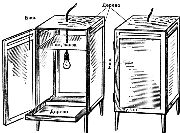
Рис. 25. Универсальная световая ловушка.
